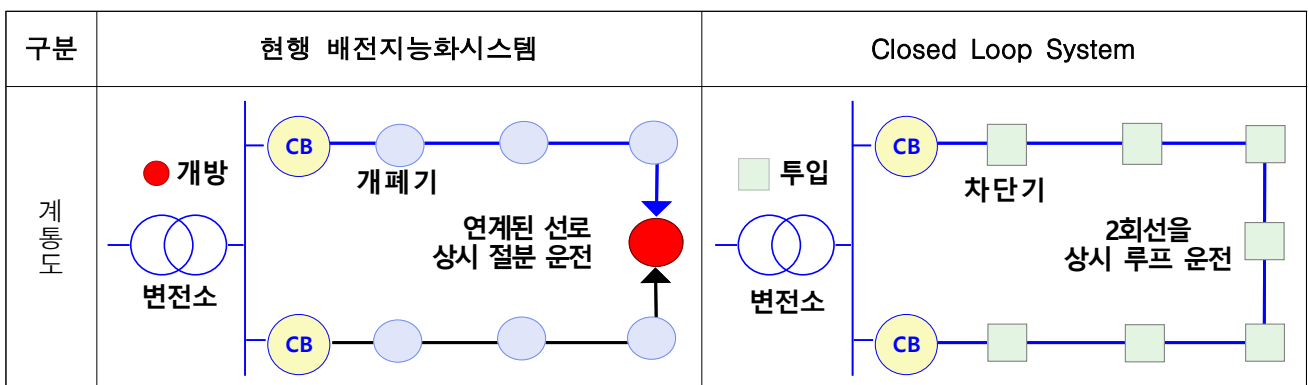
[그림 1] Closed Loop 배전계통 운전
